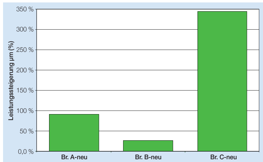
Abb. 4: Gegenüberstellung Brunnenergiebigkeiten alt / neu und Kies / Glaskugeln
